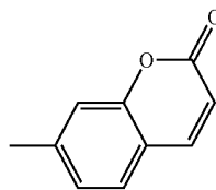
[Chem. 6]
