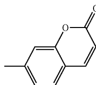
[Chem. 6]
