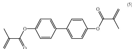
[Chem. 5]
