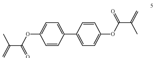
[Chem. 5]
