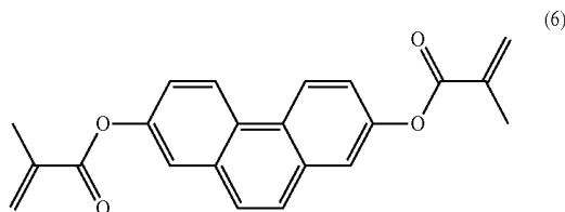
[Chem. 6]
