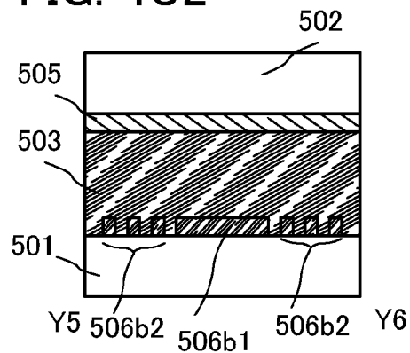
FIG. 4C2
