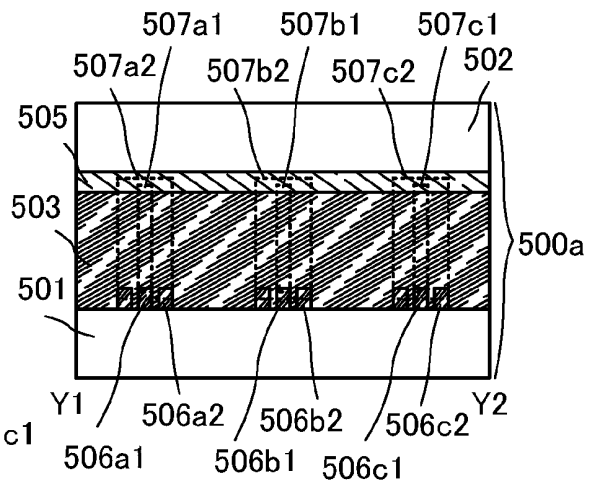
FIG. 4B2
