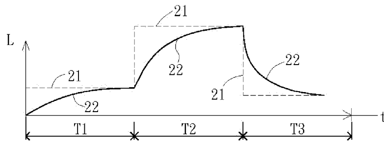
FIG. 2B(PRIOR ART)
