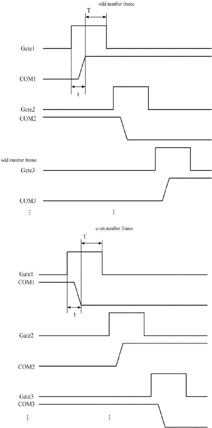
FIG.2 --Prior Art--
