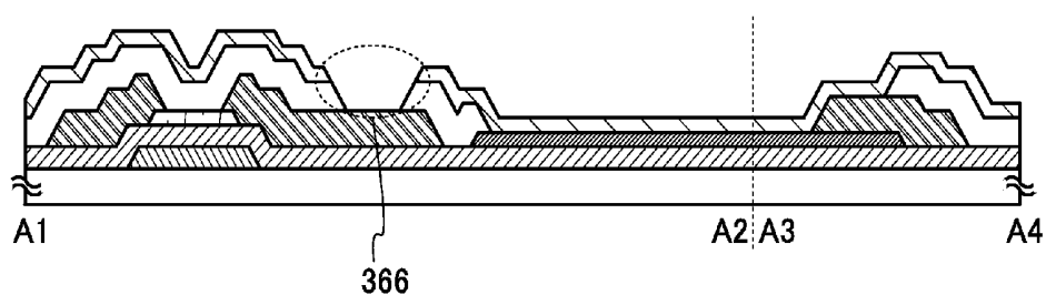
FIG. 13C
