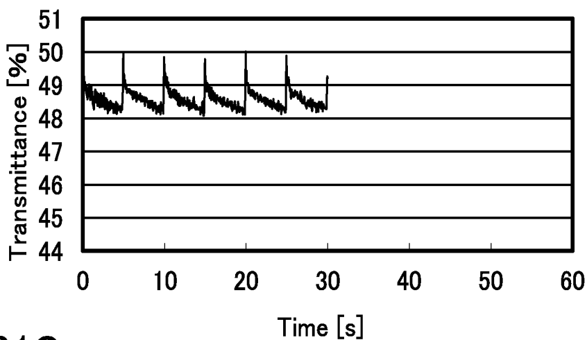
FIG. 21C
