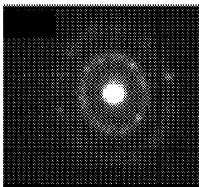
nc-OS
