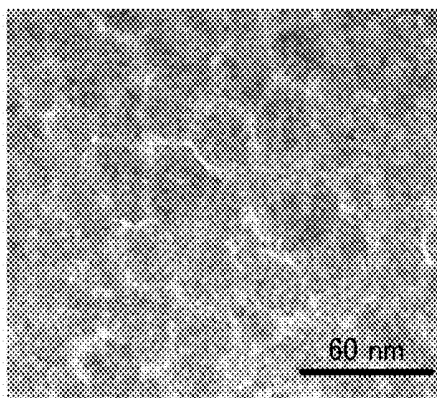
as-sputtered
