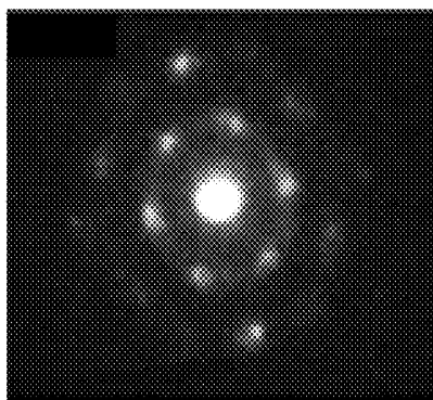
CAAC-OS
