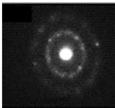
nc-OS
