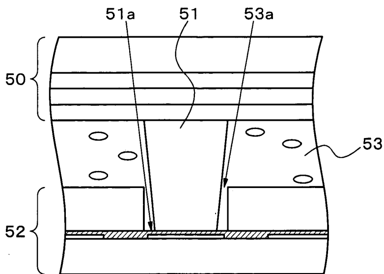
FIG. 8 ( PRIOR ART)
