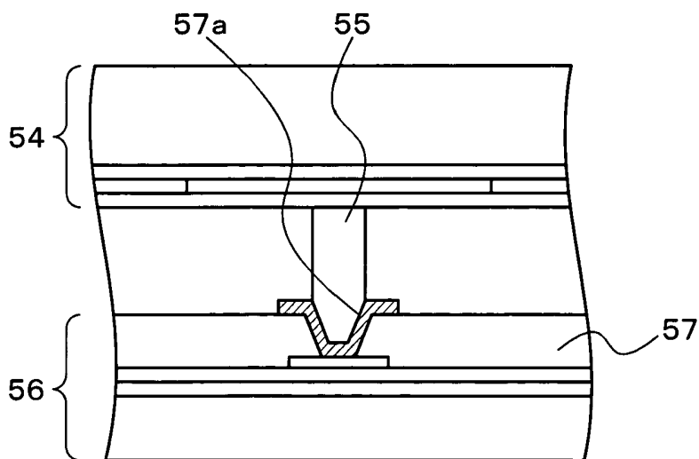
FIG. 9 ( PRIOR ART)
