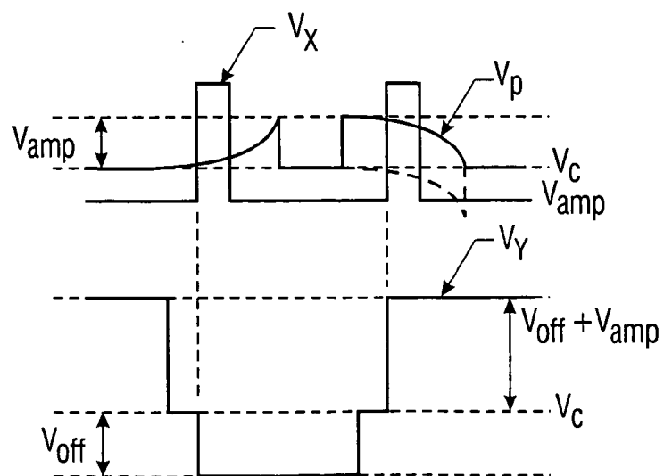
FIG. 11C
