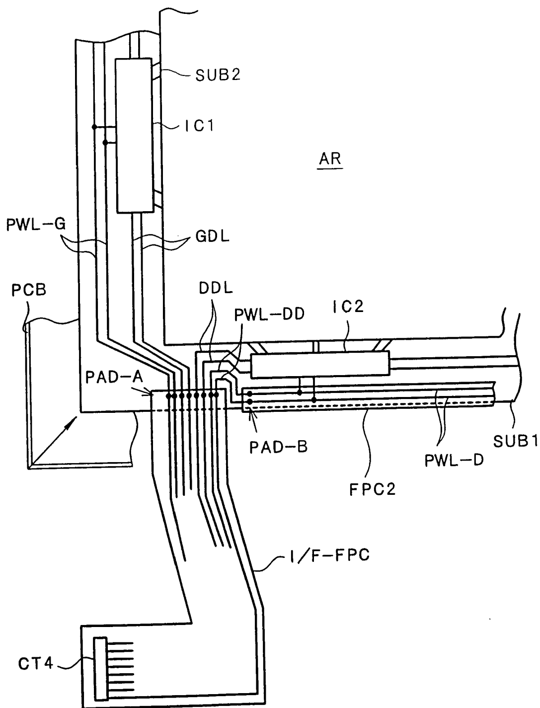
FIG. 35
