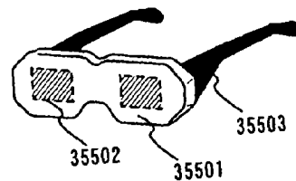
FIG. 23F
