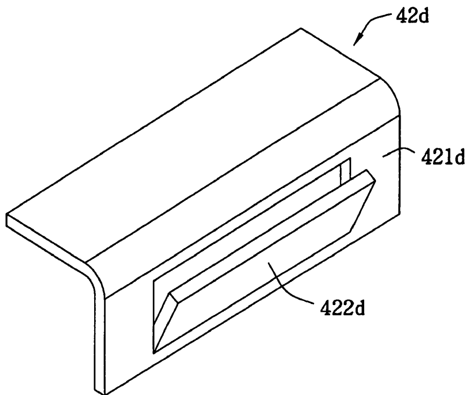
FIG. 4(e)
