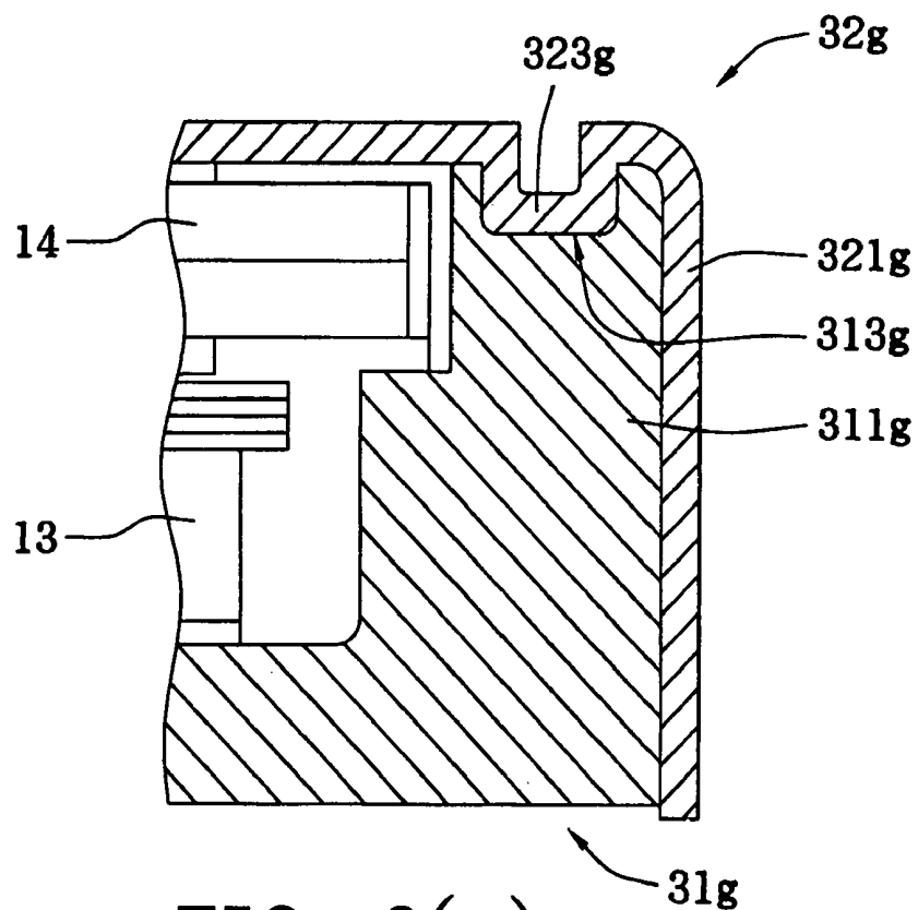
FIG. 3(g)
