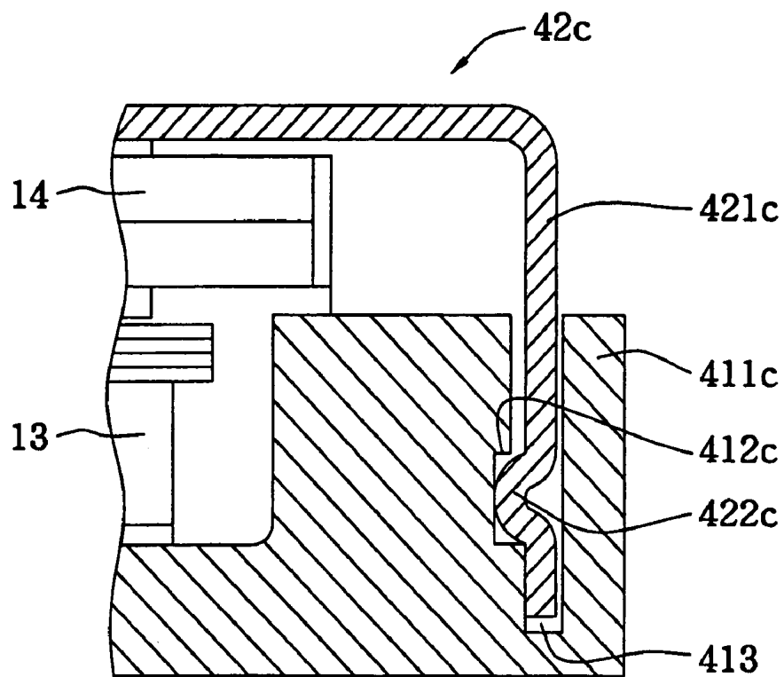
FIG. 4(c)
