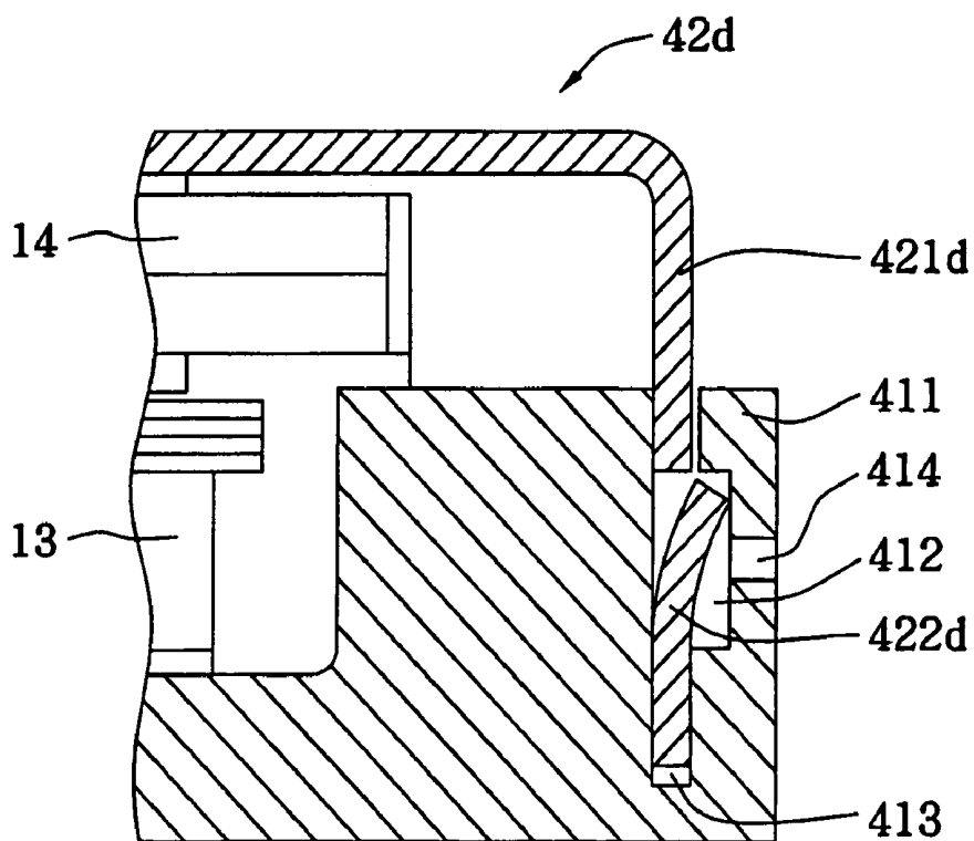
FIG. 4(d)
