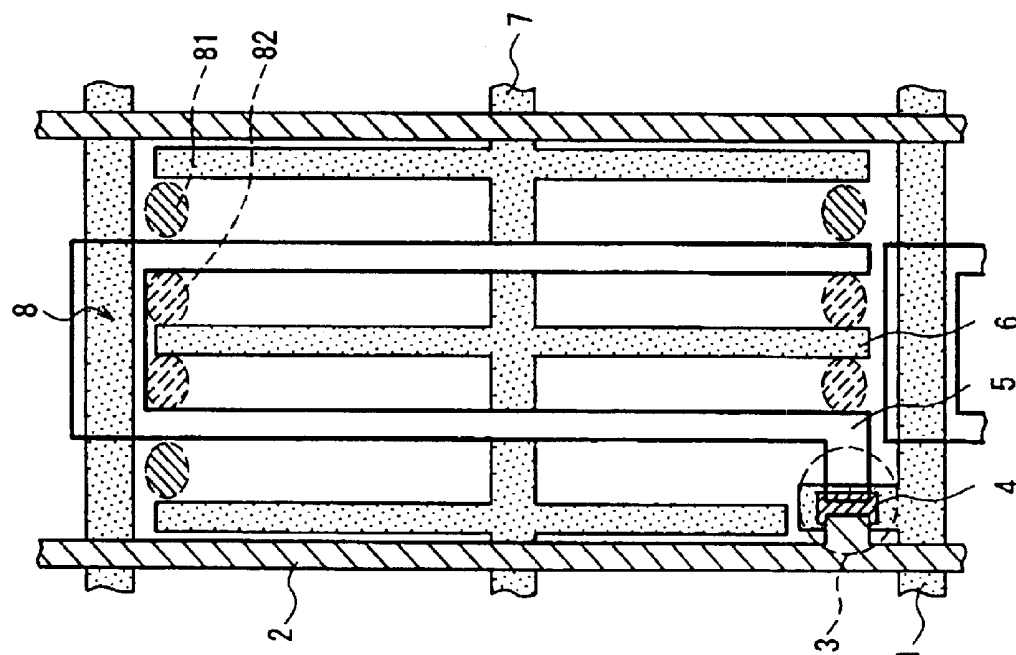
FIG. 8A (Feeding Side)
