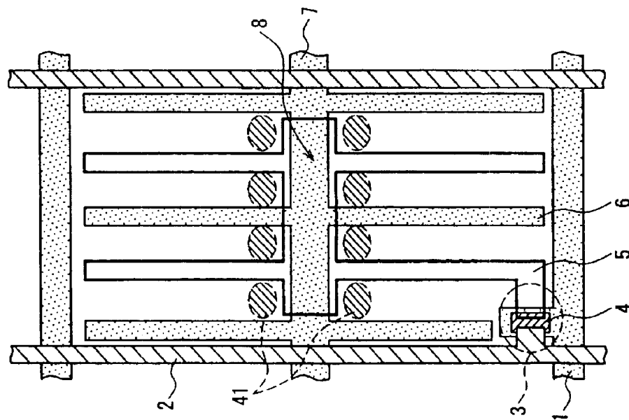
FIG. 4A (Feeding Side)
