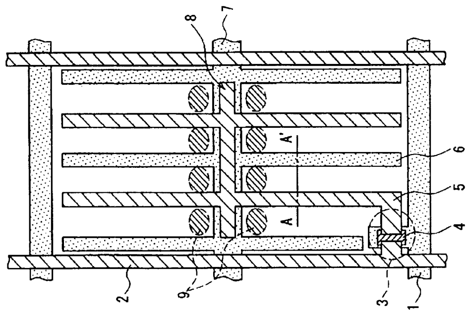
FIG. 1A (Feeding Side)
