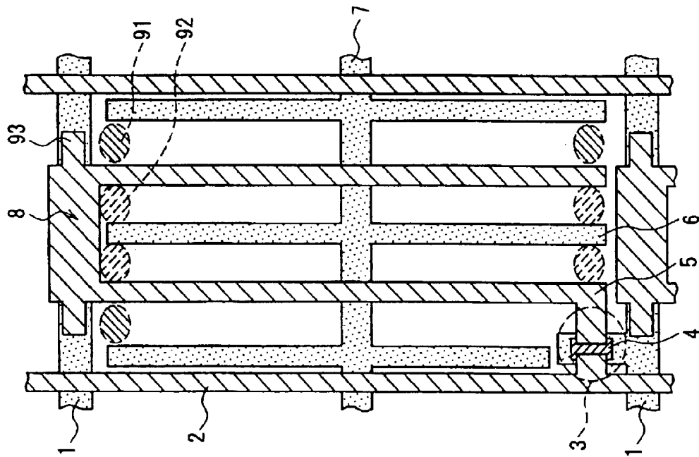
FIG. 10A (Feeding Side)
