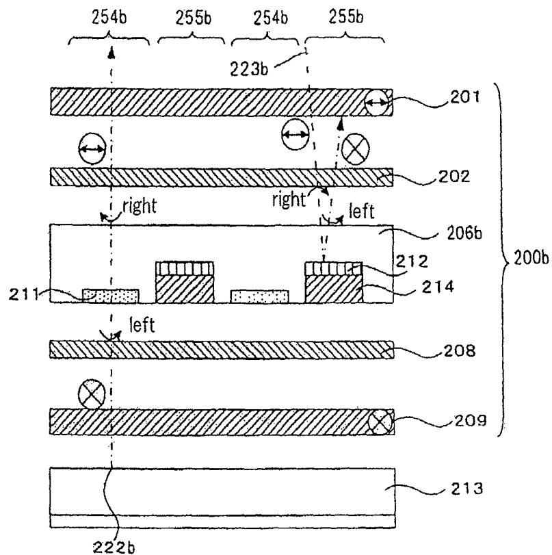
Fig.22B
