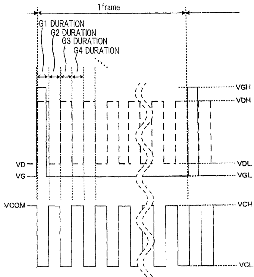
Fig.13A
