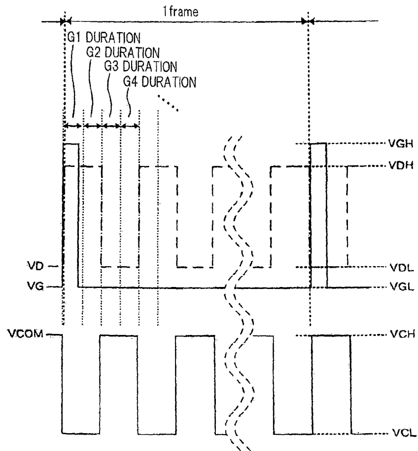
Fig.15B
