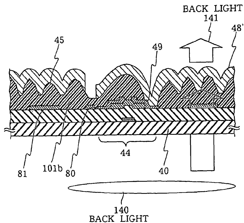
FIG. 13(b) SEMI-TRANSPARENT LIQUID CRYSTAL DISPLAY APPARATUS
