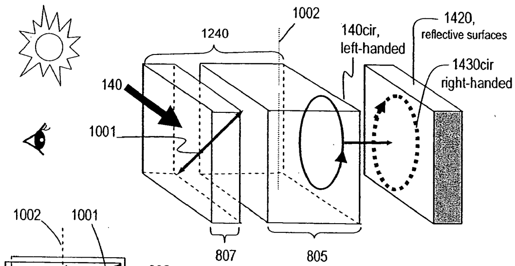
FIG. 14A
