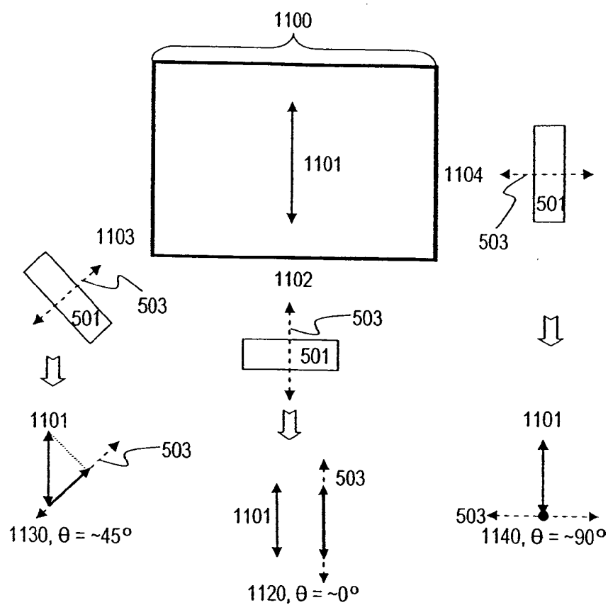
FIG. 11A
