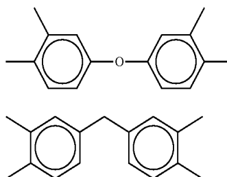
[Chem 5]
