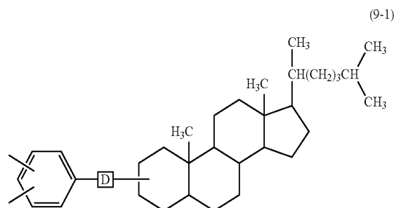
[Chem 9]
