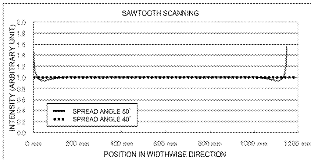
FIG. 15C
