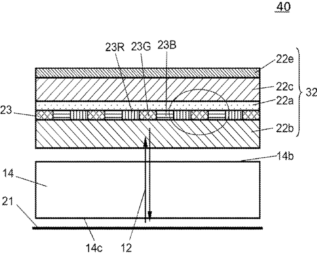
FIG. 12A
