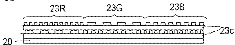
FIG. 5D
