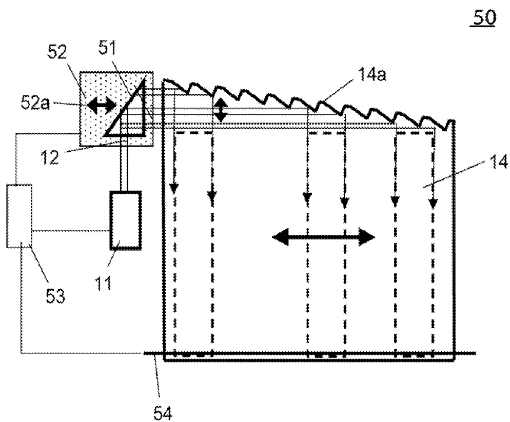
FIG. 14C
