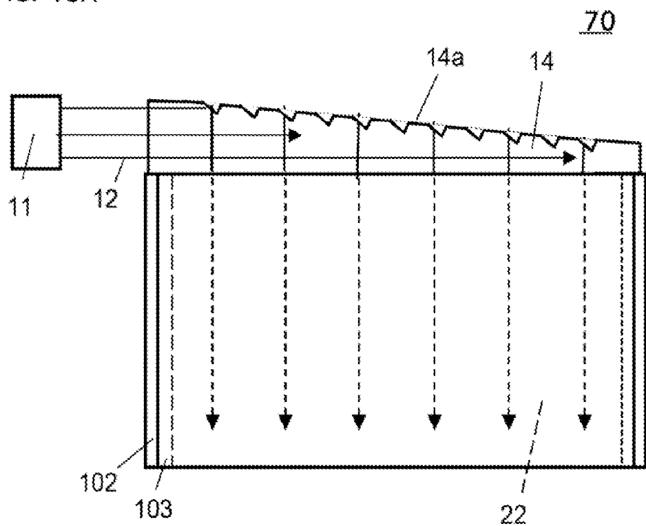
FIG. 18A
