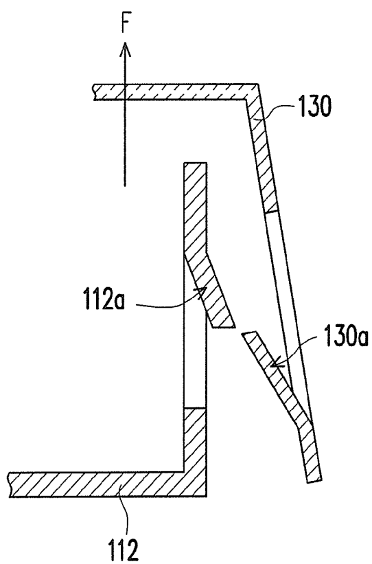
FIG. 2B(PRIOR ART)
