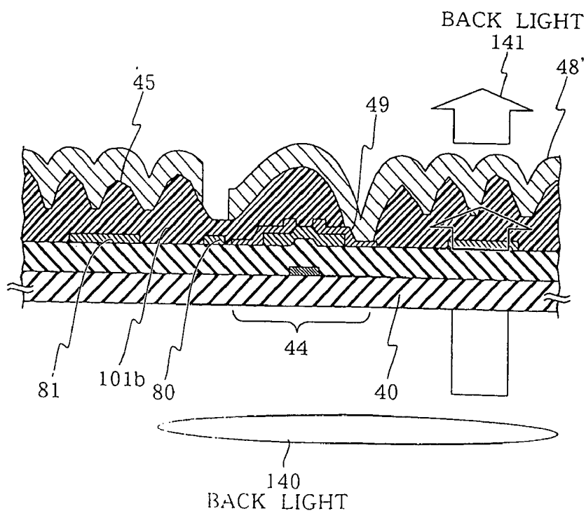
FIG. 13(b) SEMI-TRANSPARENT LIQUID CRYSTAL DISPLAY APPARATUS
