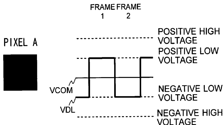
Fig. 21A PRIOR ART
