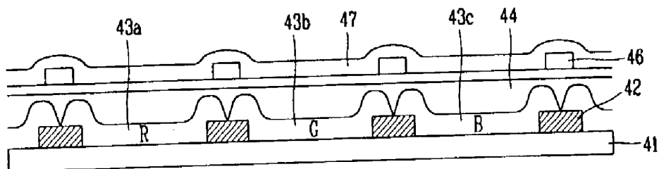
FIG. 4F
