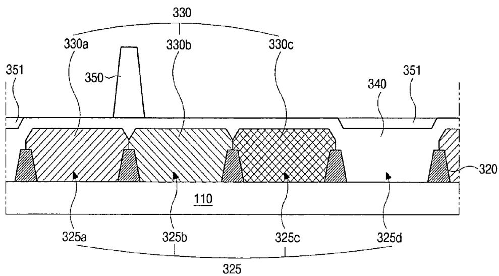
FIG. 5H
