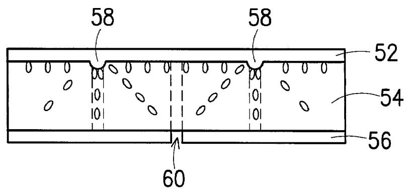
FIG. 1B(PRIOR ART)
