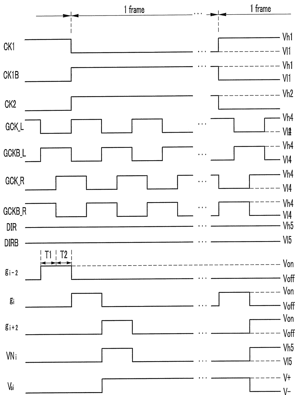
FIG.17B
