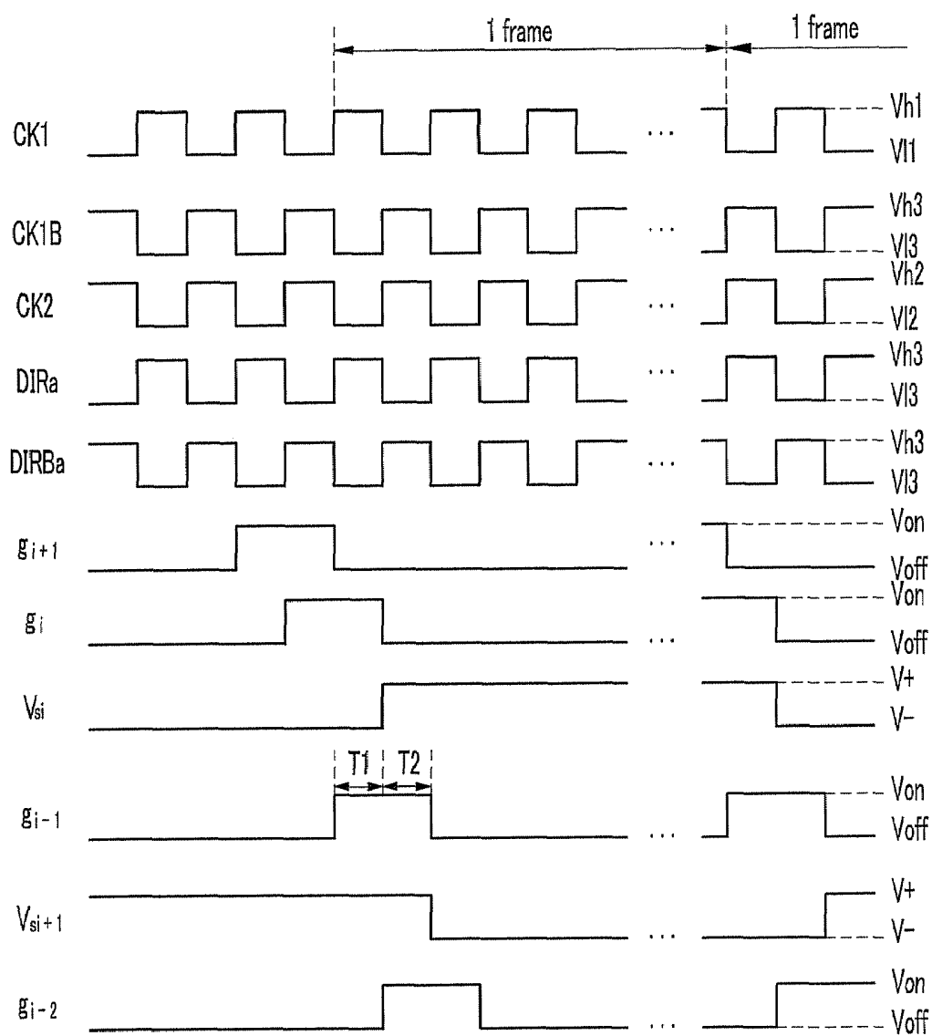
FIG.8B
