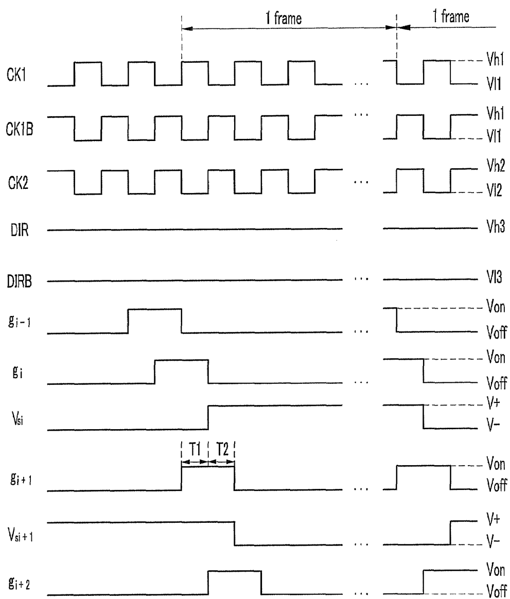
FIG. 7A
