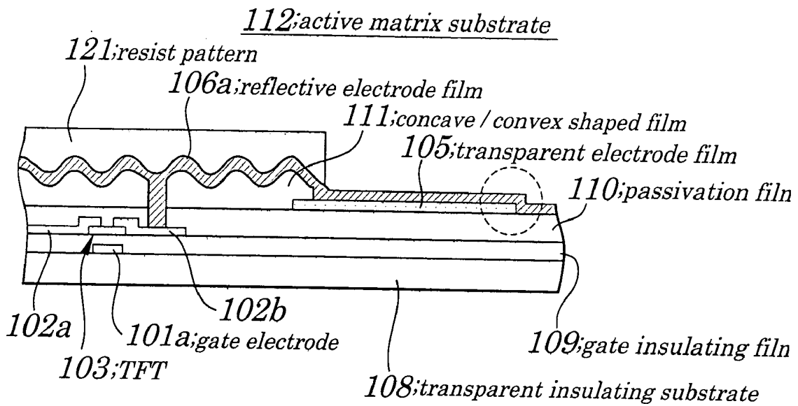
FIG. 31B(PRIOR ART)
