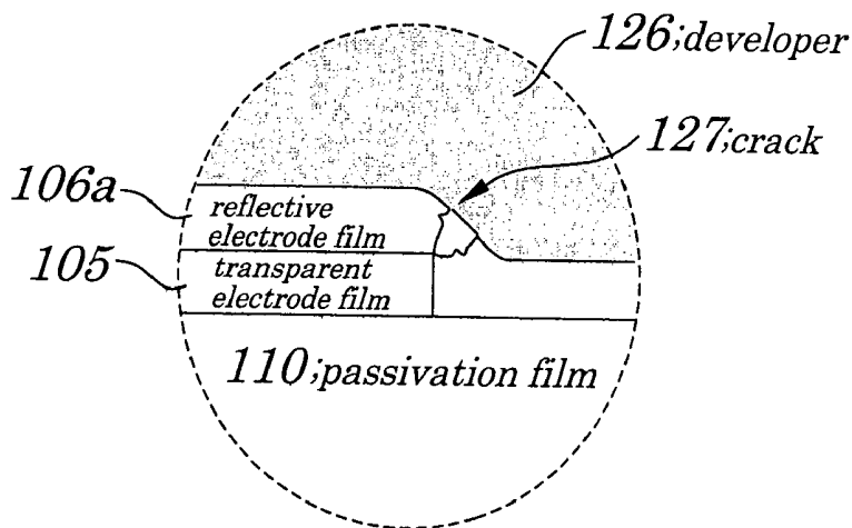
FIG. 31B(PRIOR ART)
