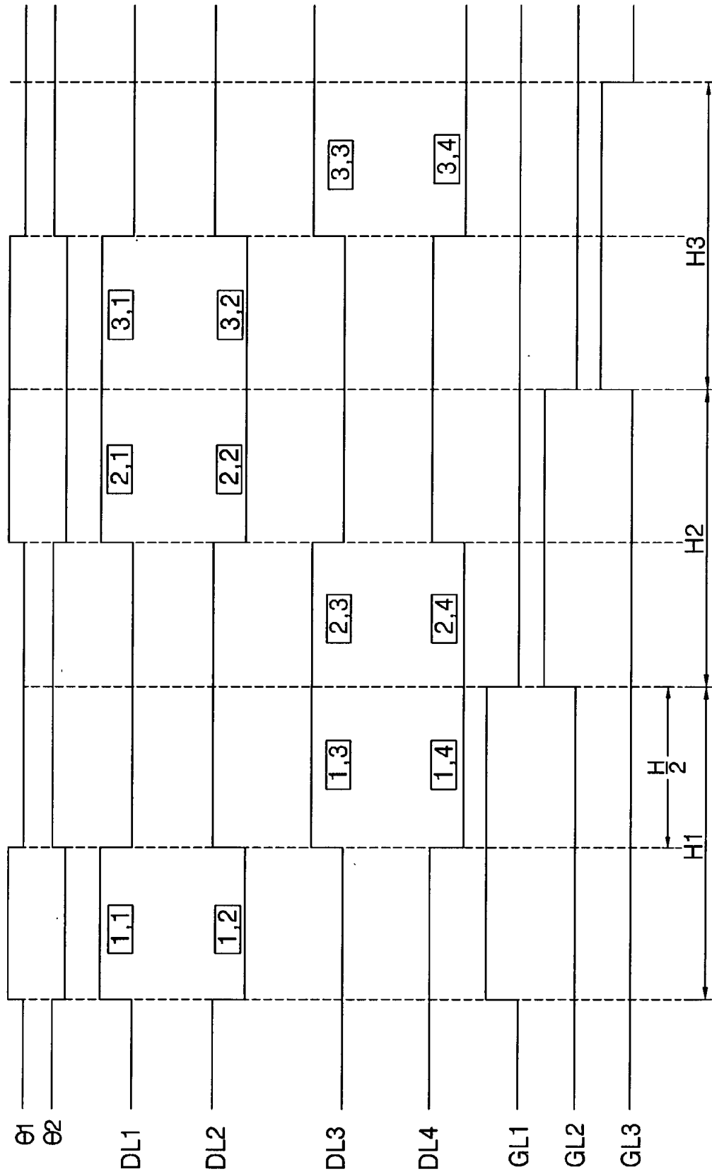
FIG. 16A
