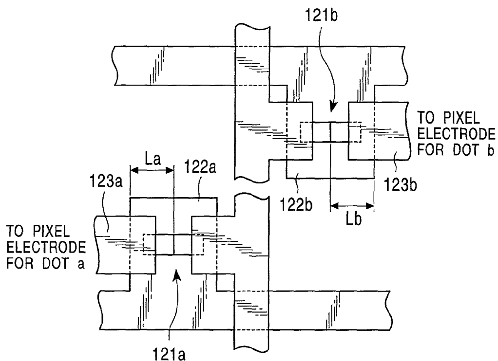
FIG. 25A
