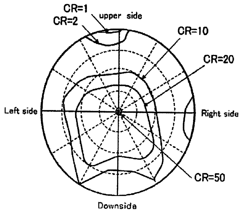
FIG.2B(PRIOR ART)
