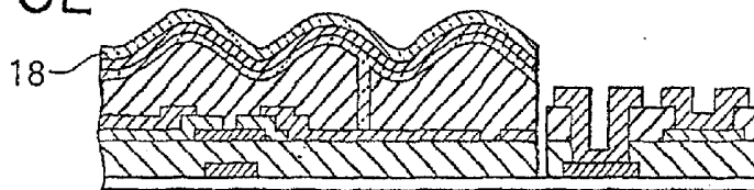
FIG. 15F
