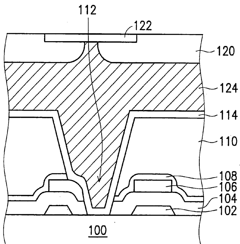
FIG. 4E
