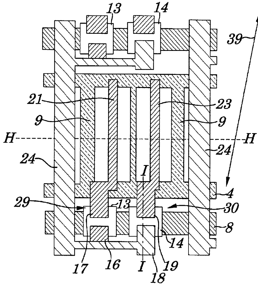
FIG. 30
