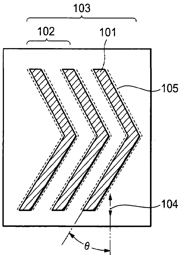
FIG. 2B(PRIOR ART)
