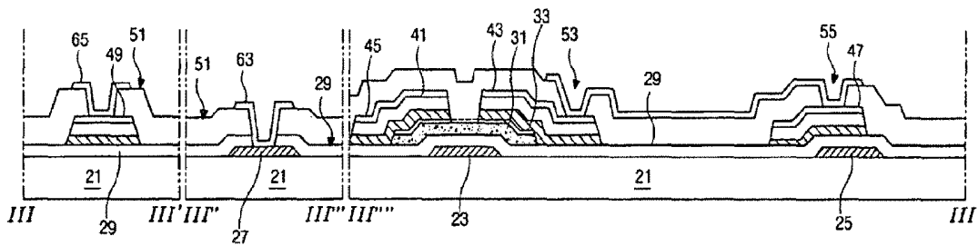
(related art) FIG. 4E
