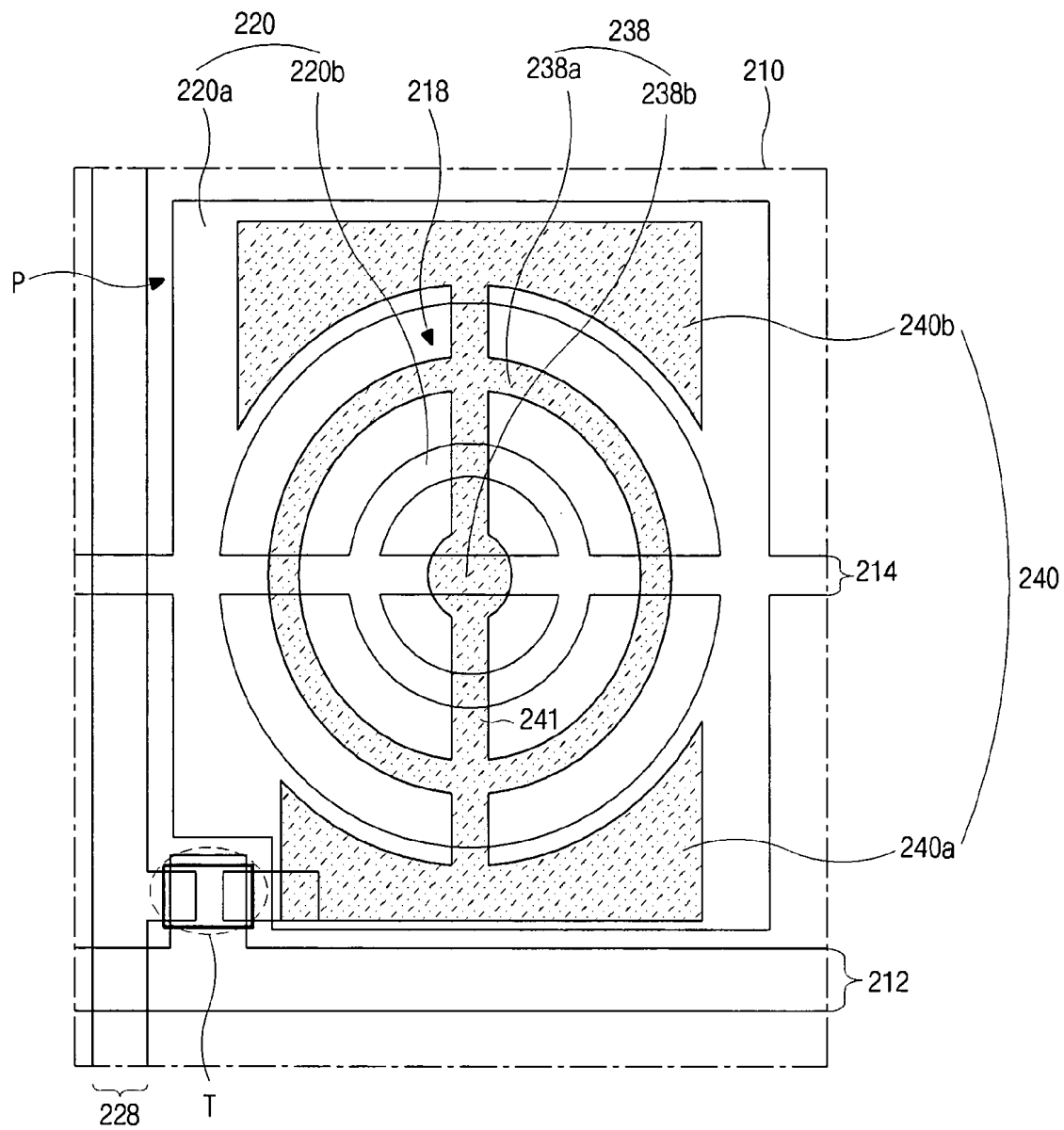
FIG. 7A
