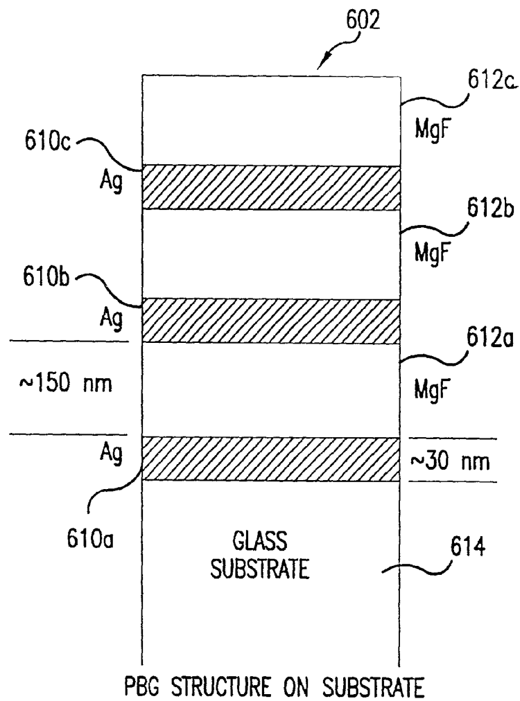
FIG. 6A
