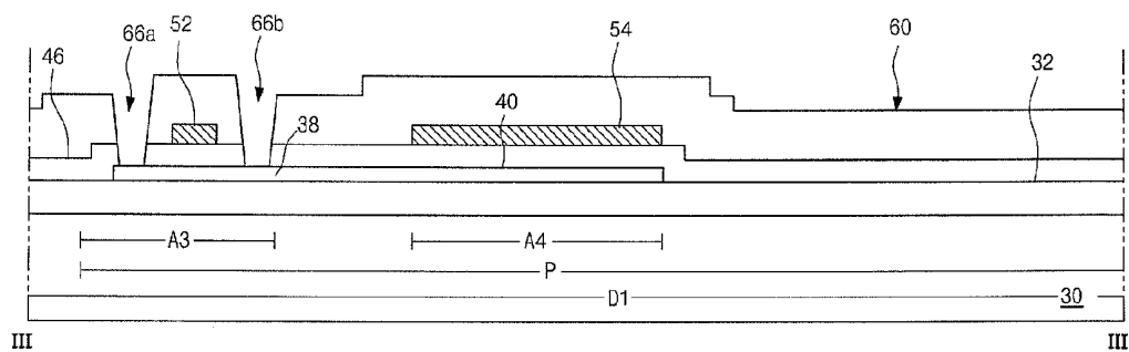
FIG. 6F PRIOR ART
