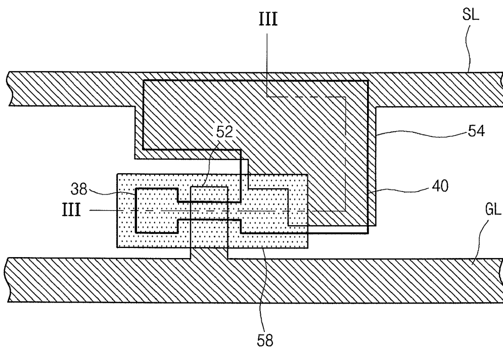
FIG. 5E PRIOR ART
