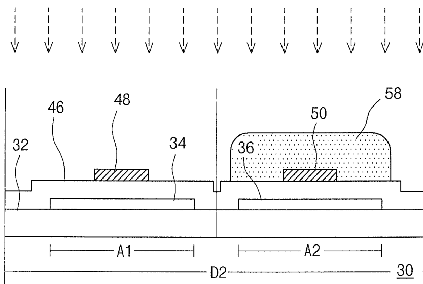
FIG. 4E PRIOR ART p + ion doping
