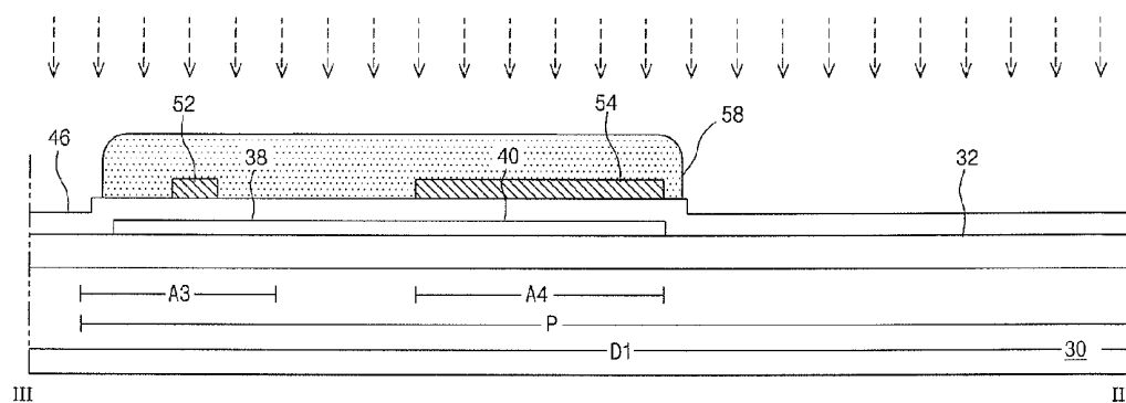
FIG. 6E PRIOR ART
