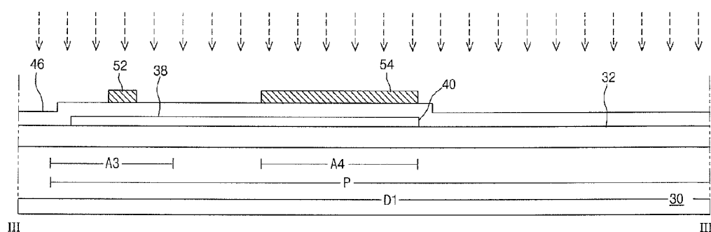
FIG. 6E PRIOR ART
