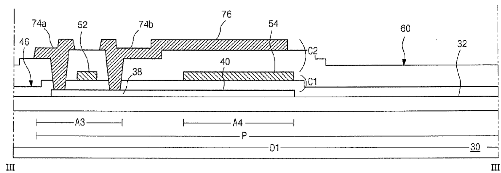
FIG. 6G PRIOR ART
