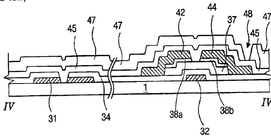
FIG. 4E (RELATED ART)
