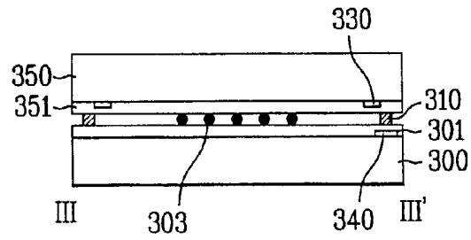
FIG. 6C
