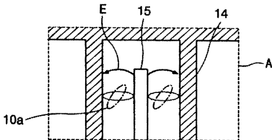
(prior art) FIG. 9A
