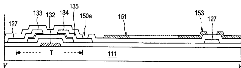
FIG. 11C
