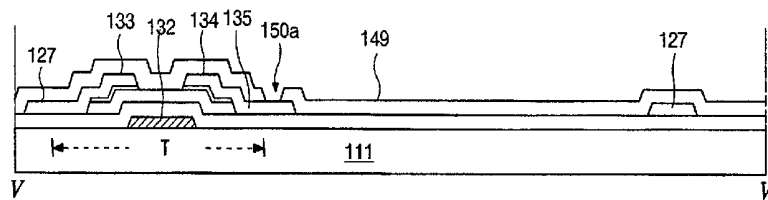
FIG. 11B
