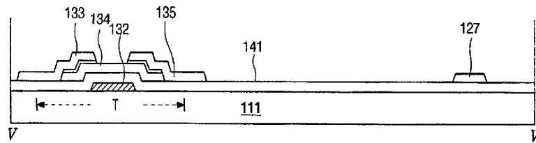
FIG. 11A
