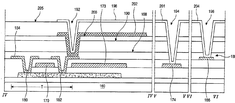
FIG. 13F
