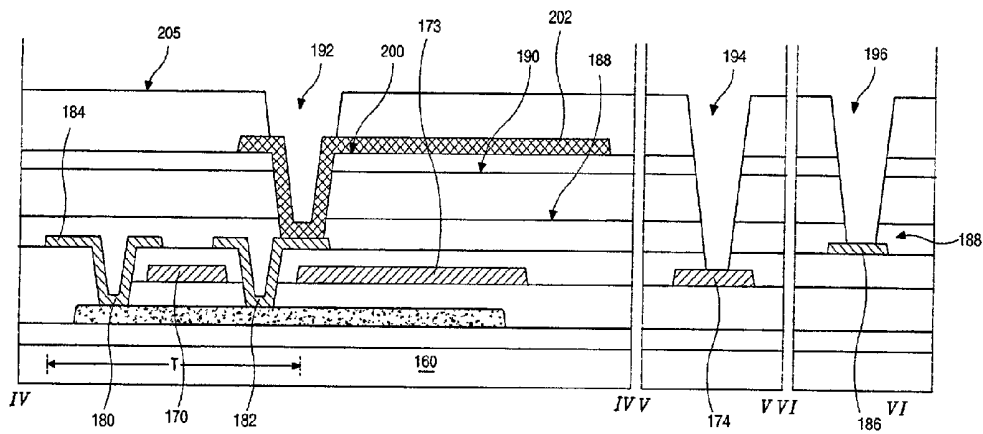
FIG. 13E
