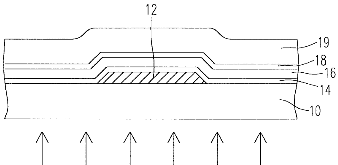
Fig. 1B(PRIOR ART)
