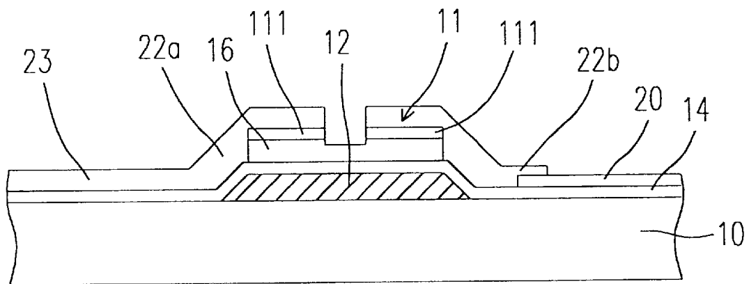
Fig. 1E(PRIOR ART)
