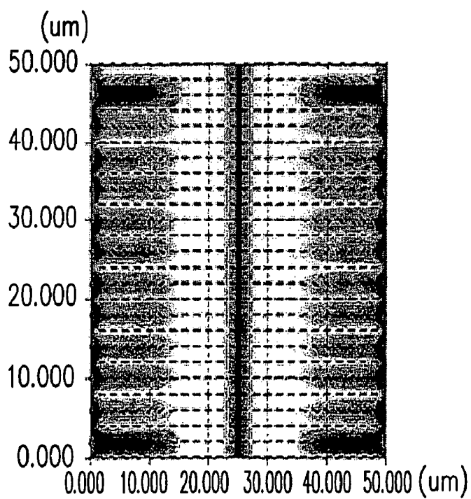
FIG. 2B(PRIOR ART)
