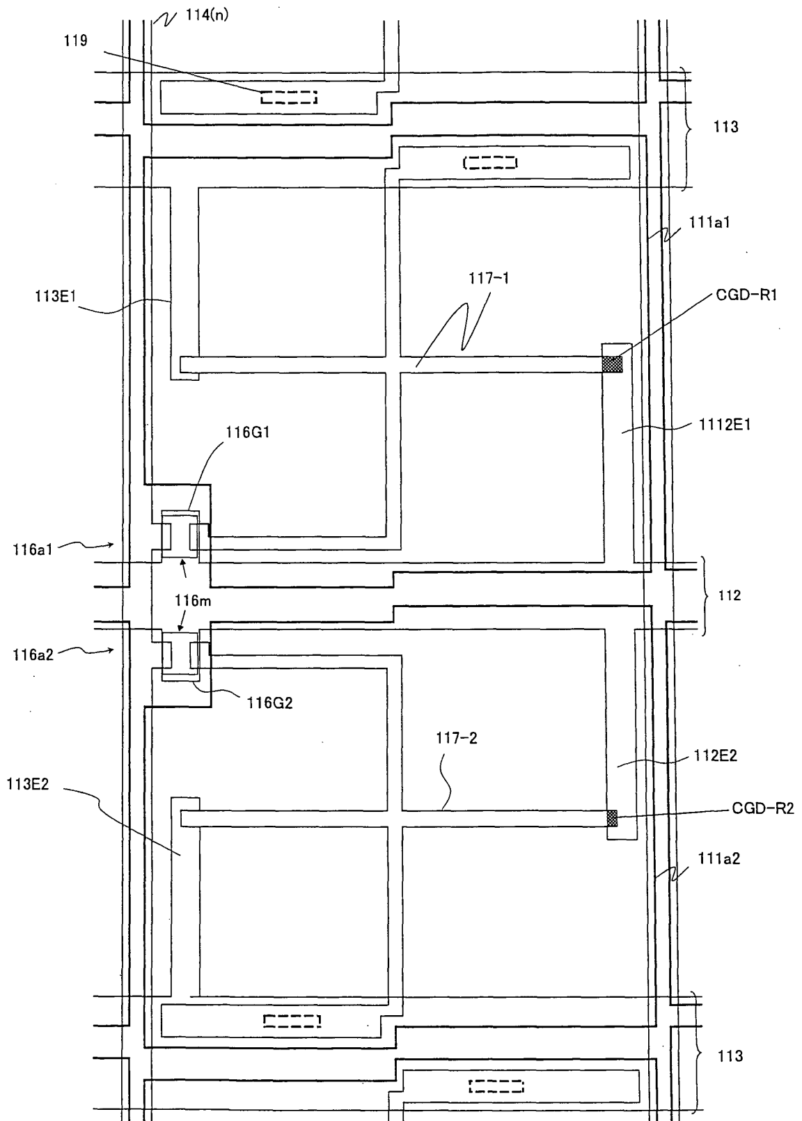
FIG. 29
