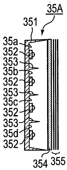
FIG. 4B
