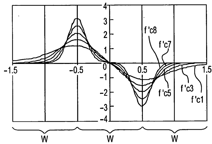
FIG. 31B
