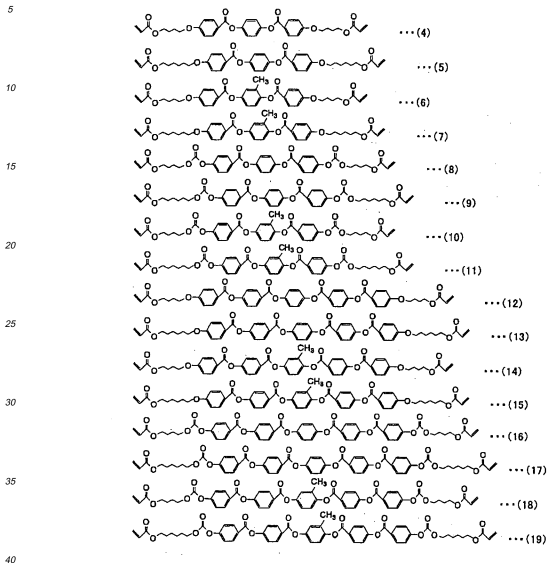
[Chem 6]
