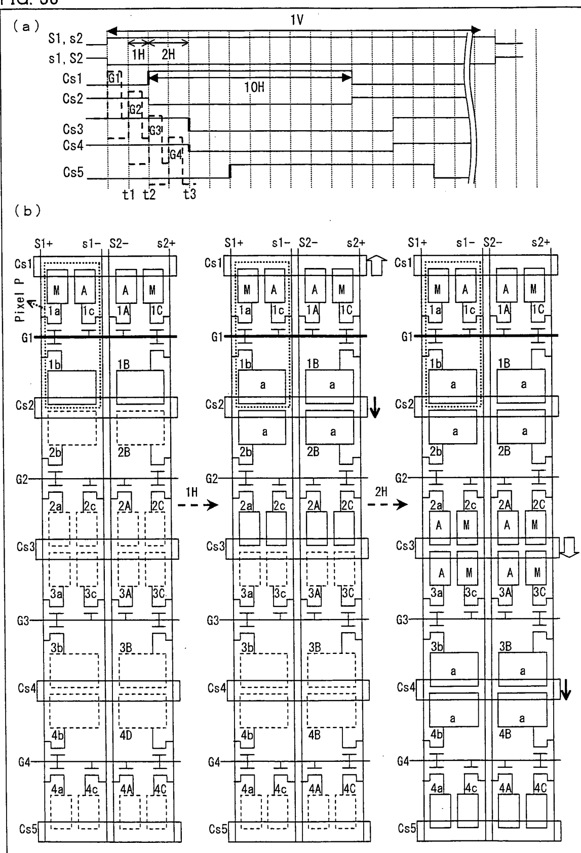
FIG. 36
