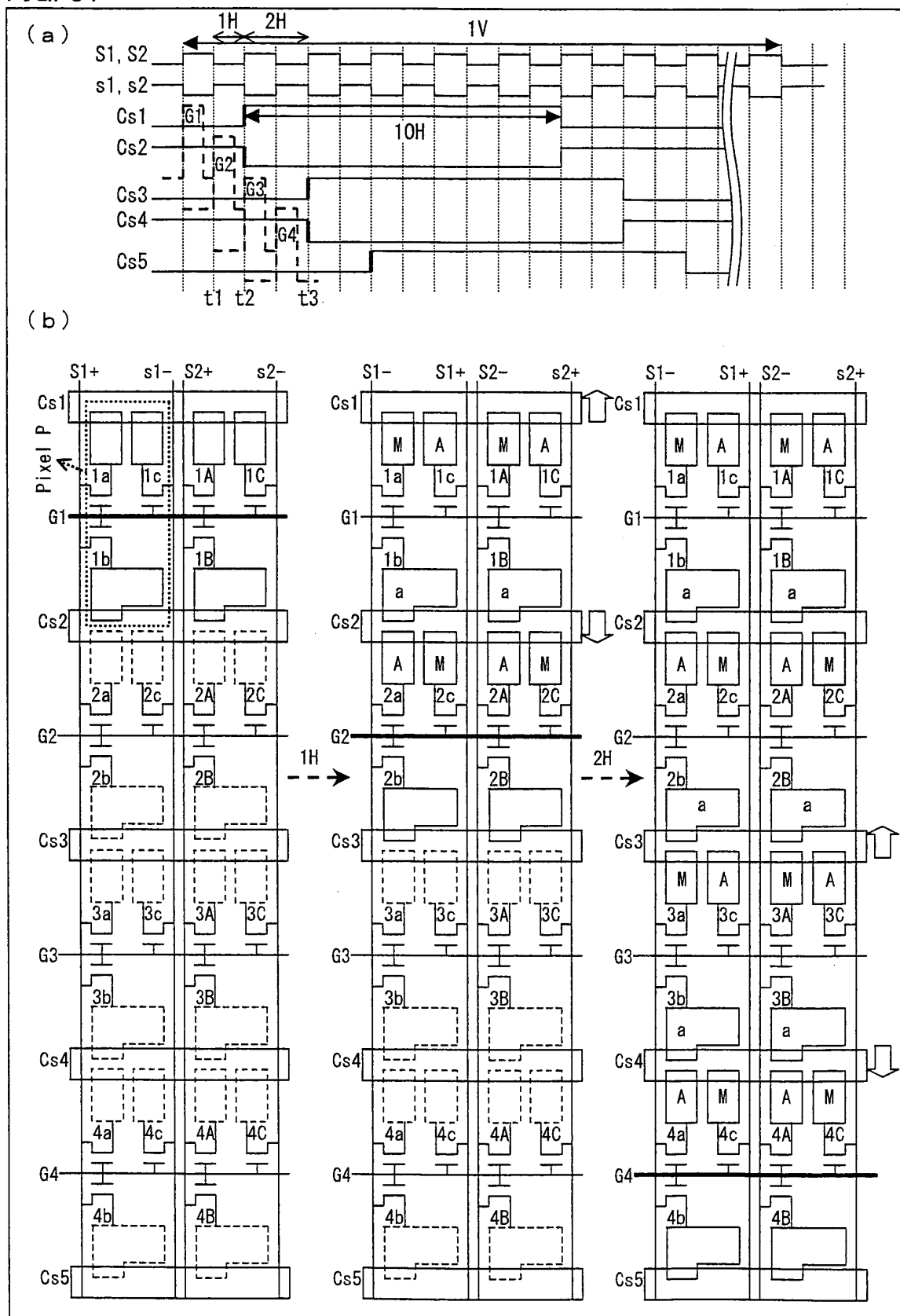
FIG. 31
